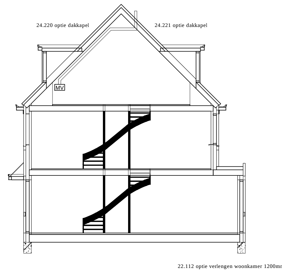
doorsnede
