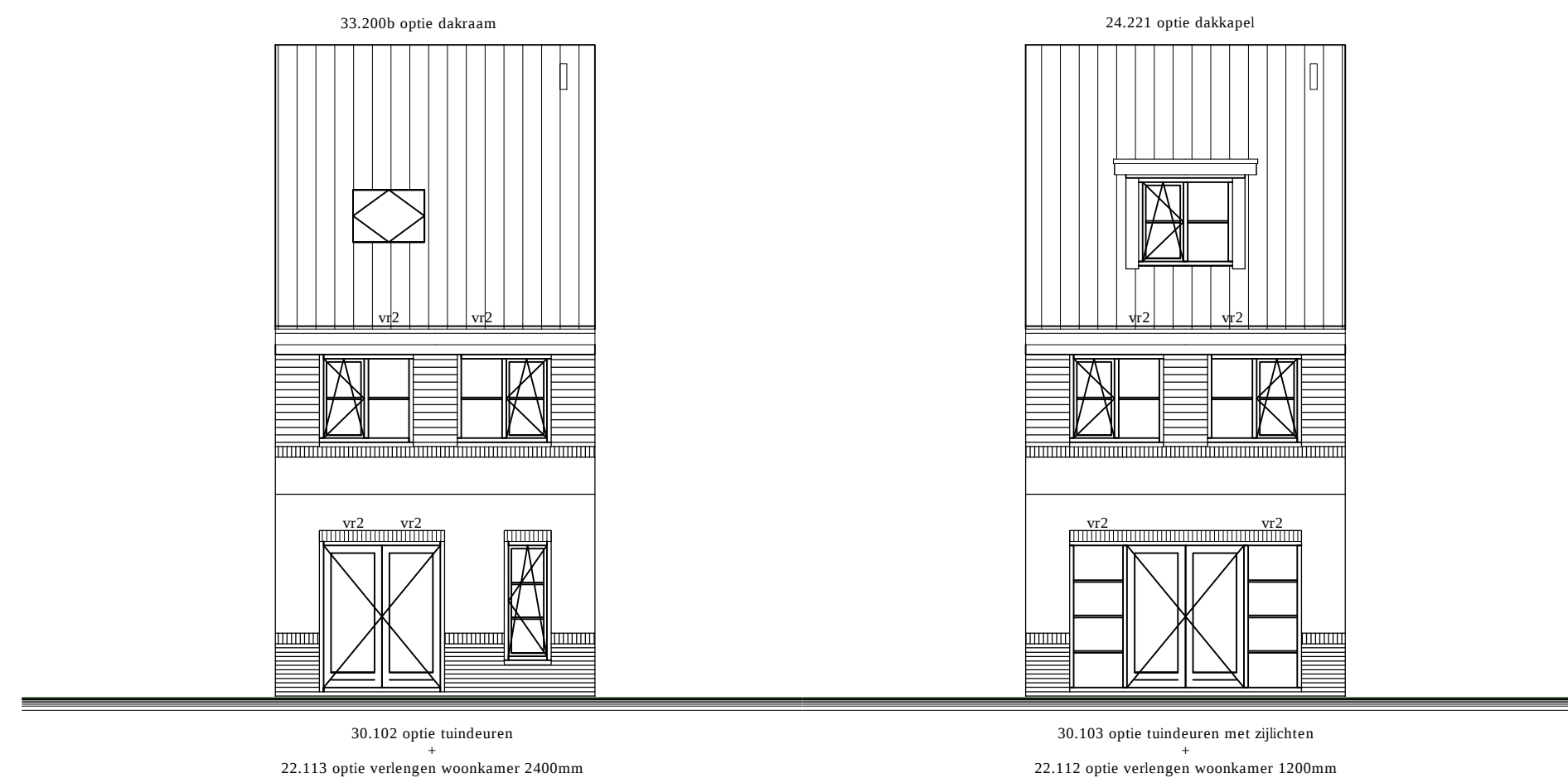
achtergevel
