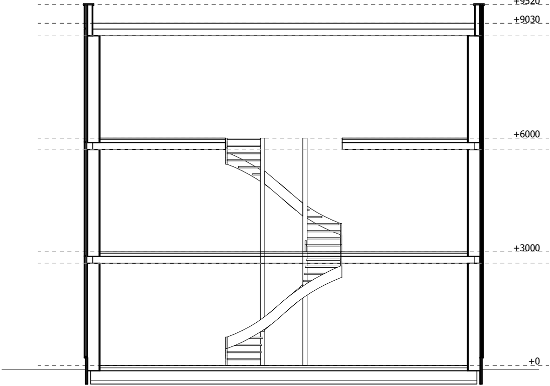
langsdoorsnede
