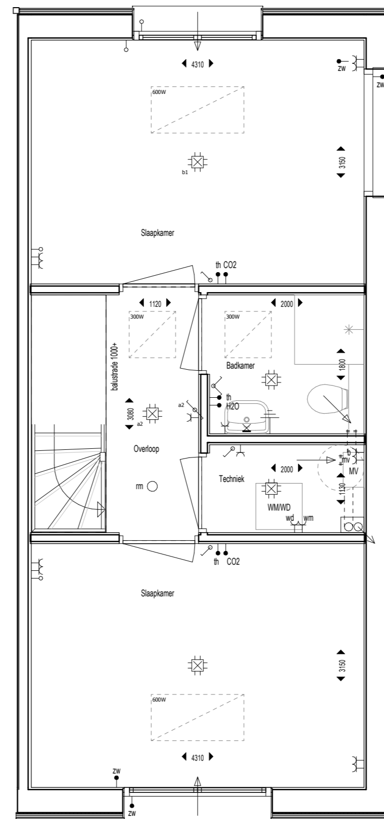
tweede verdieping
