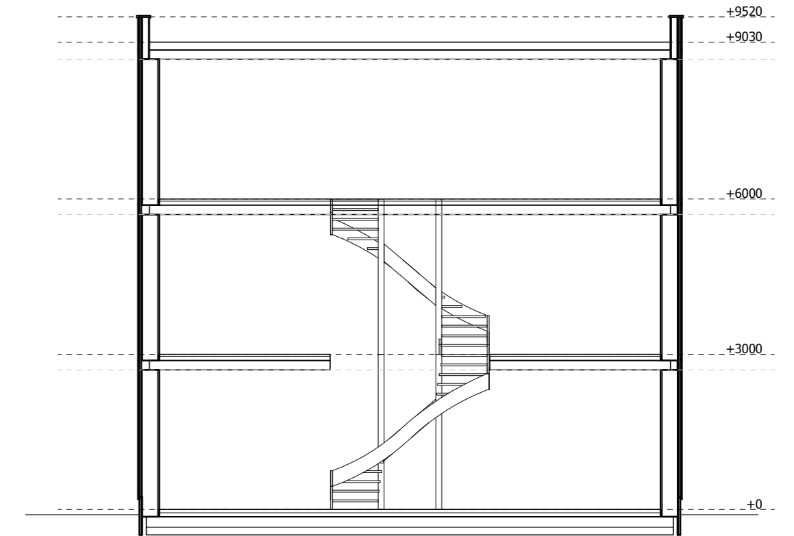
langdoorsnede
