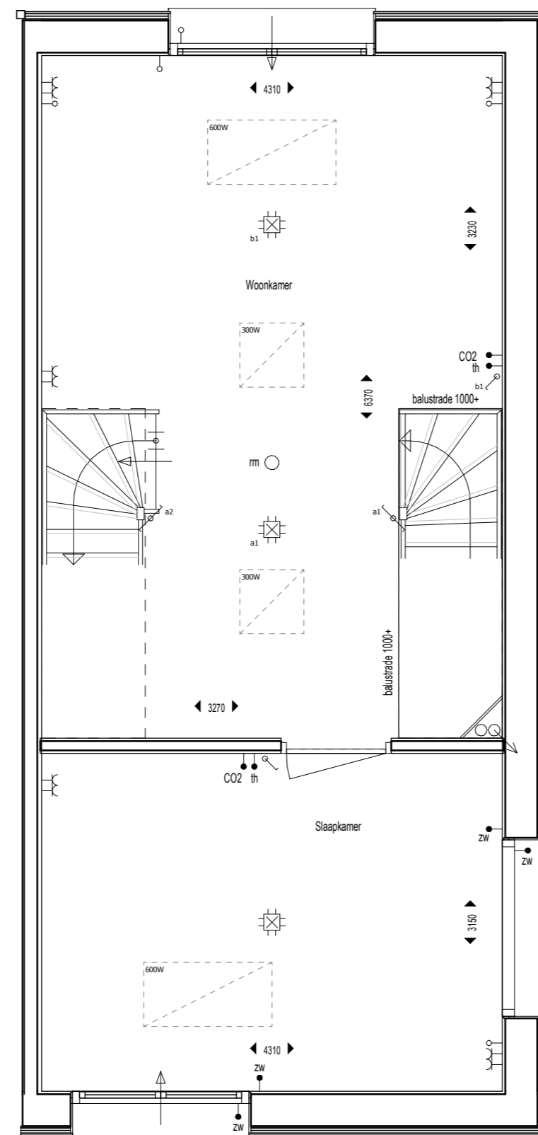
eerste verdieping
