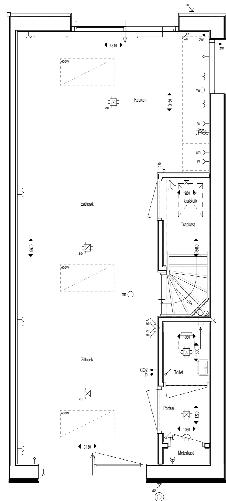
begane grond
