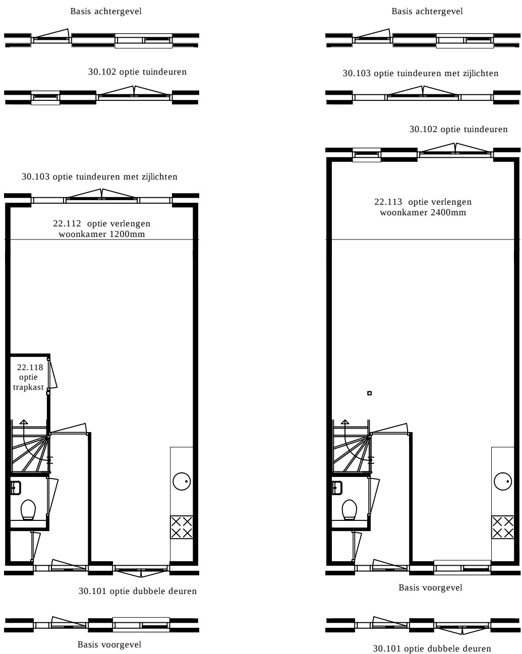
begane grond
