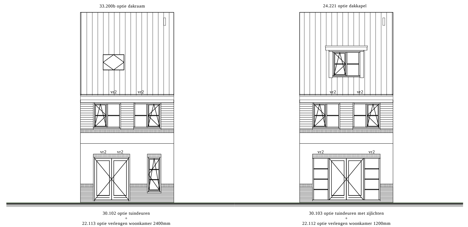
achtergevel
