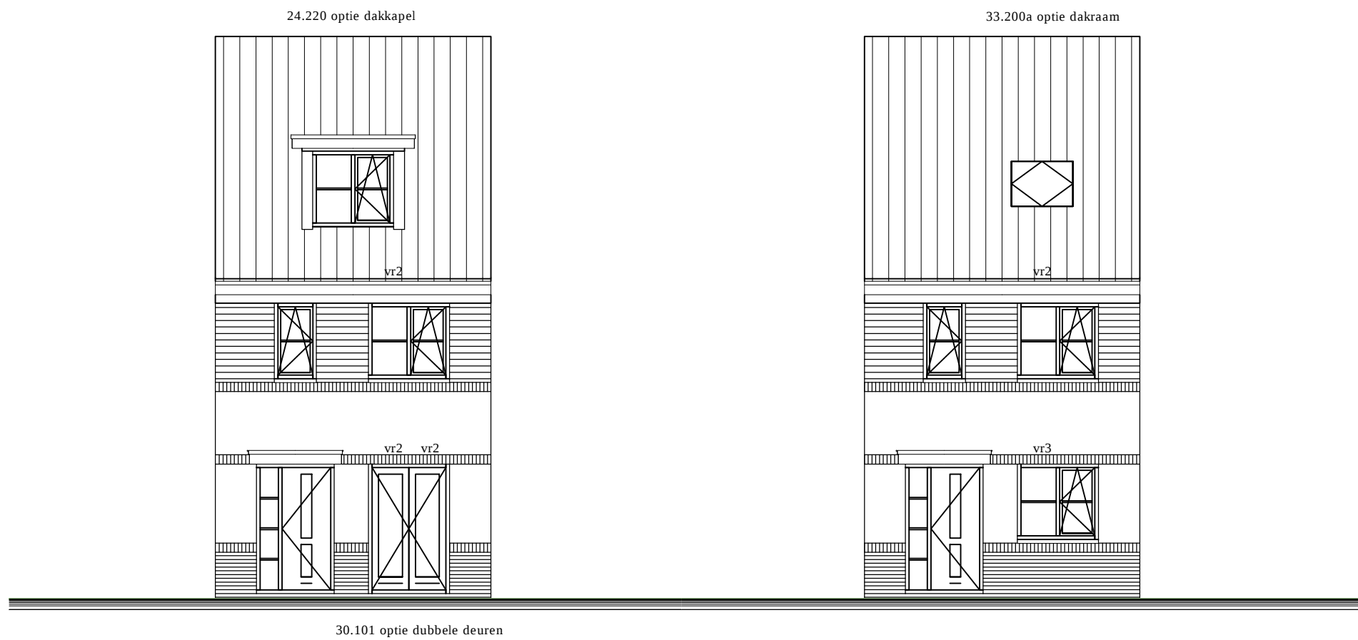
voorgevel
