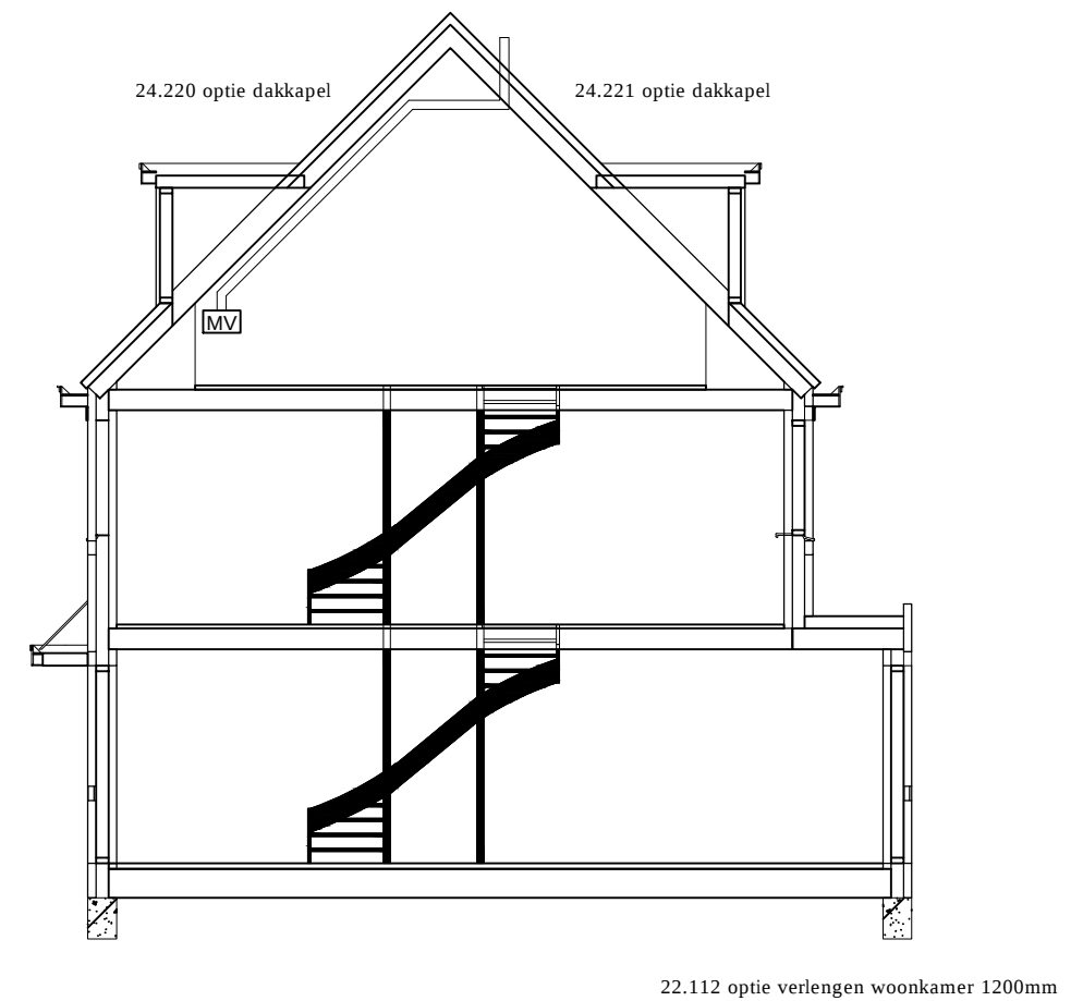
doorsnede
