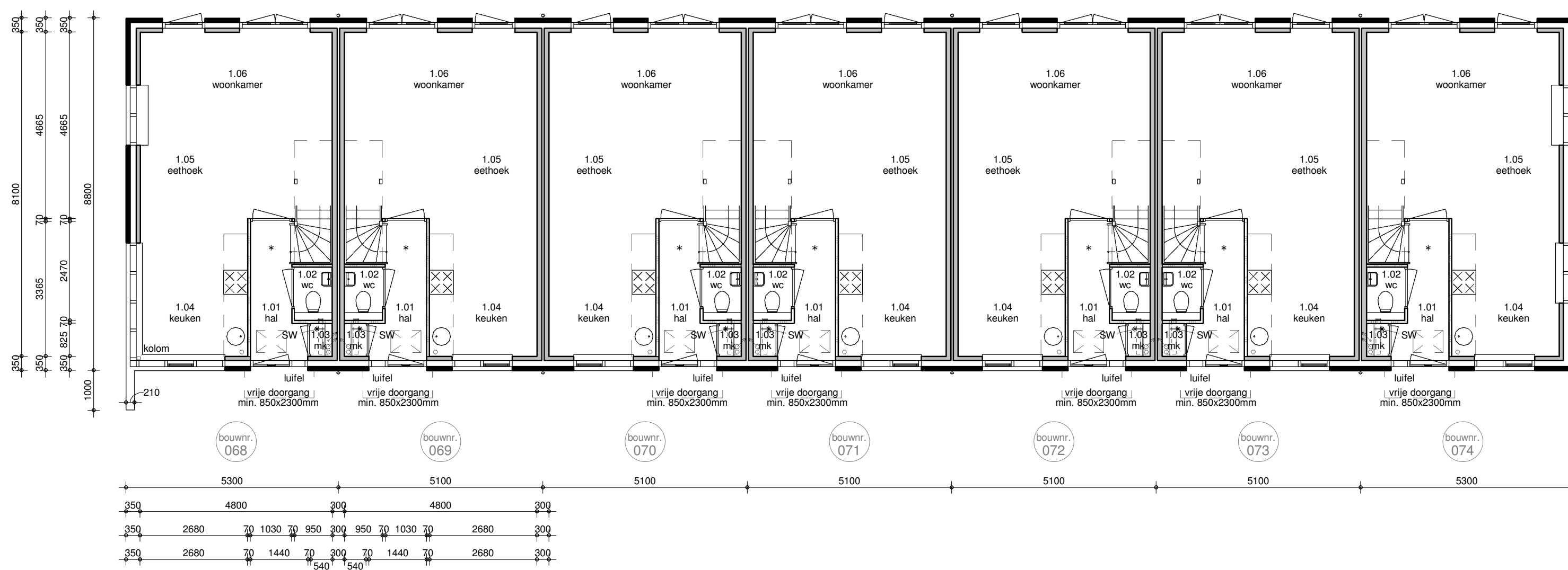
begane grond
