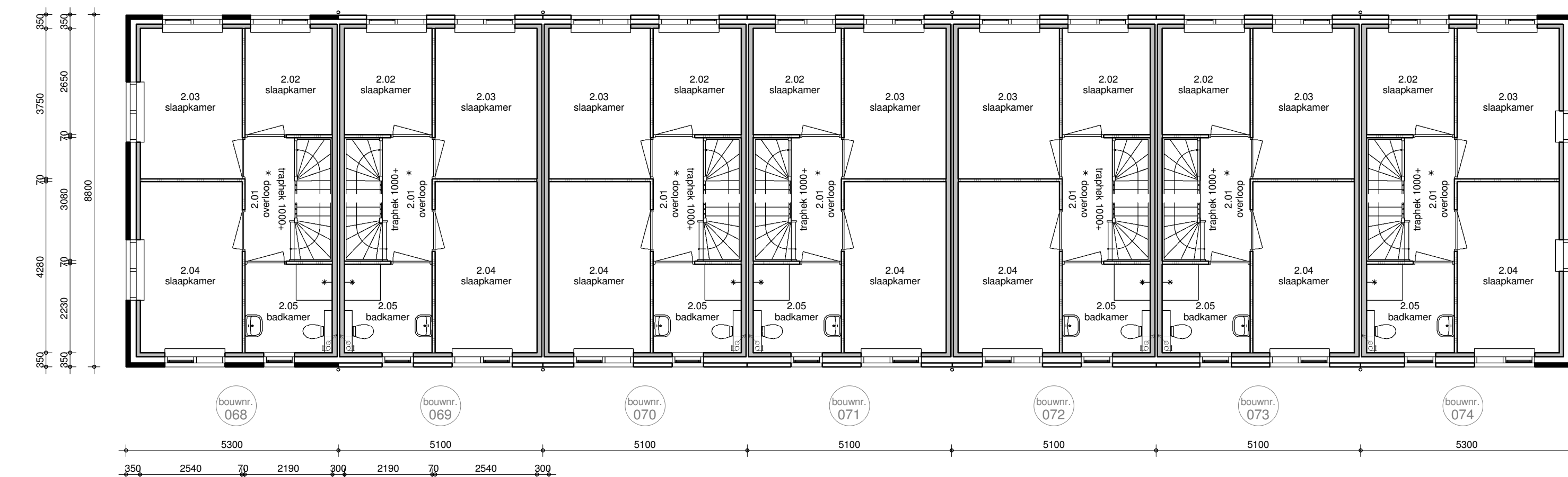
eerste verdieping
