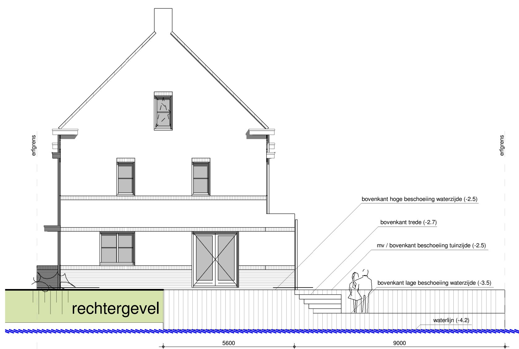
achtergevel
