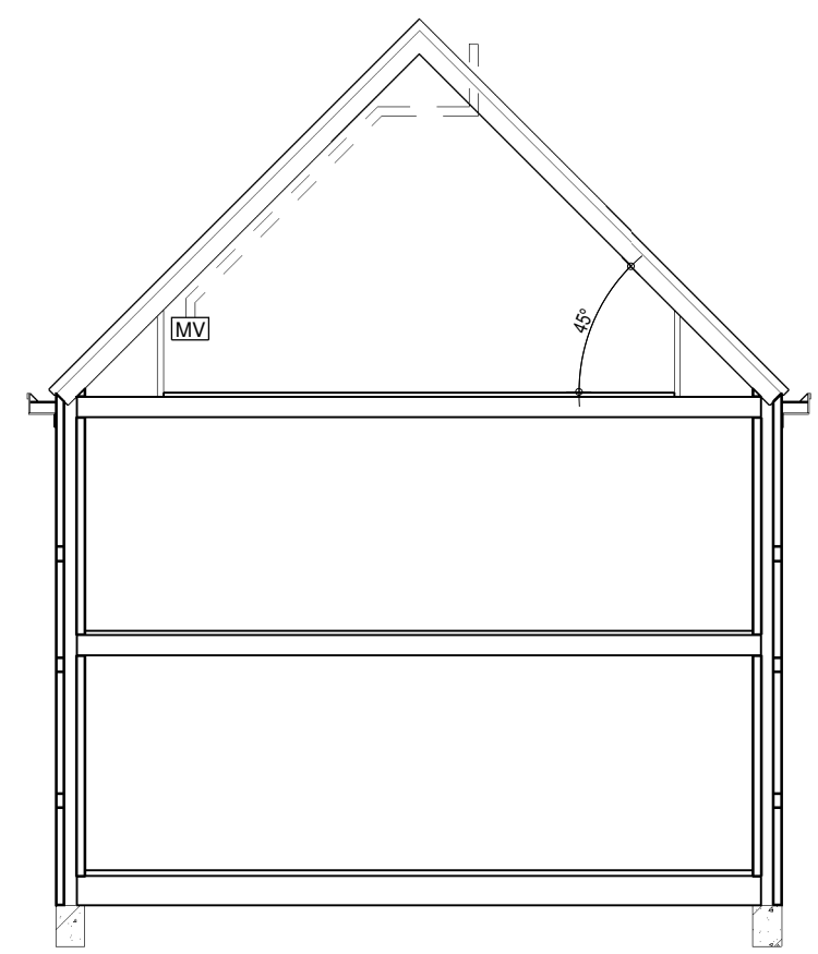
doorsnede
