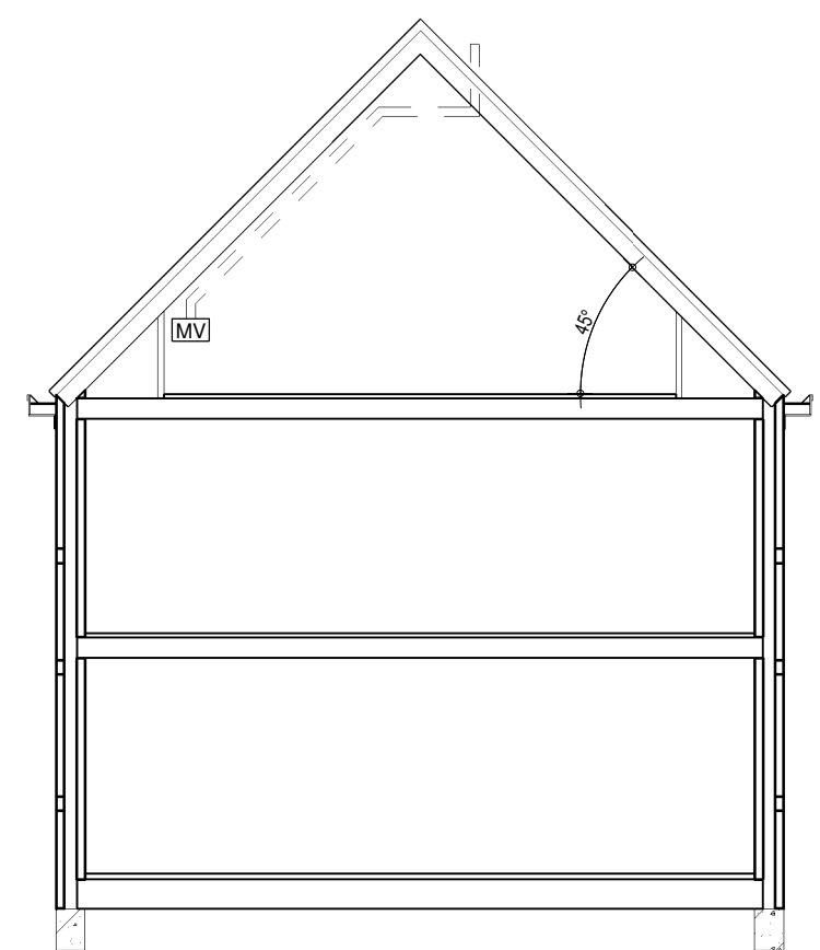
doorsnede
