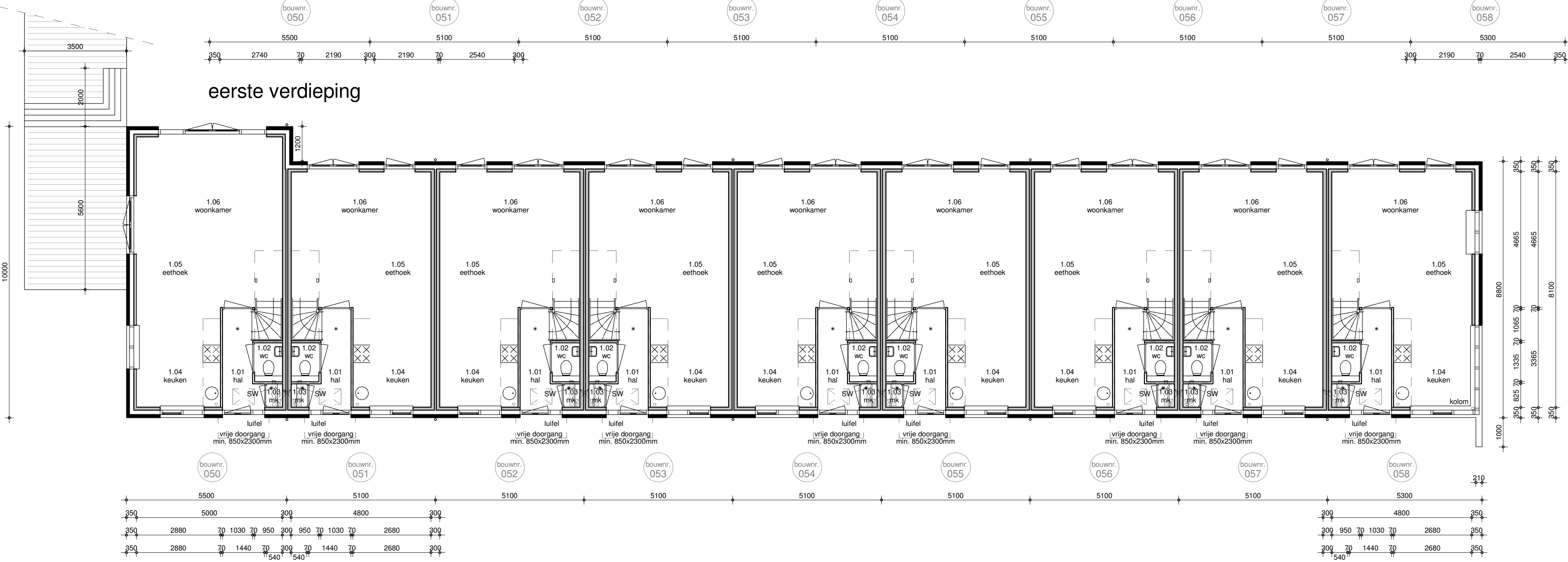
begane grond
