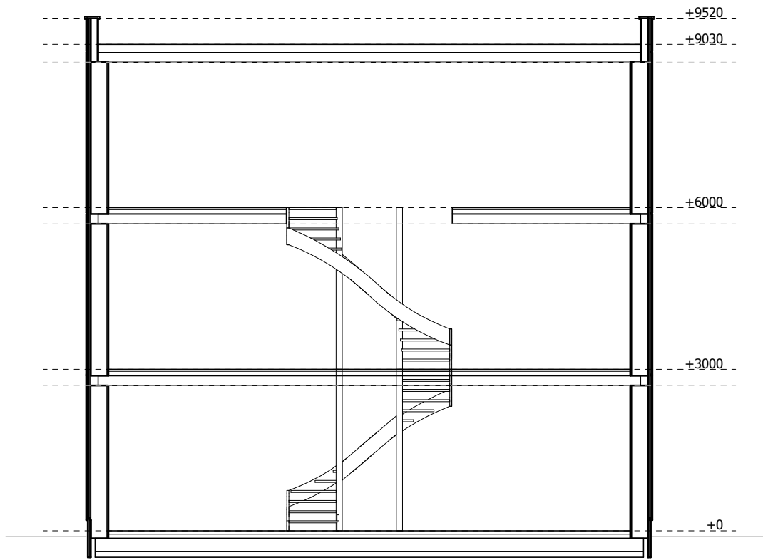
langsdoorsnede
