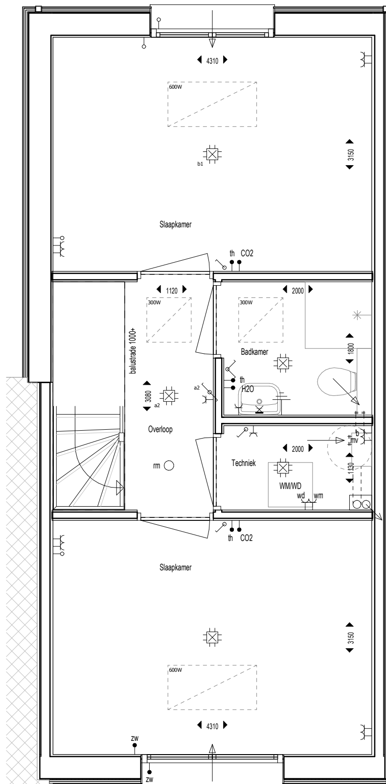
tweede verdieping
