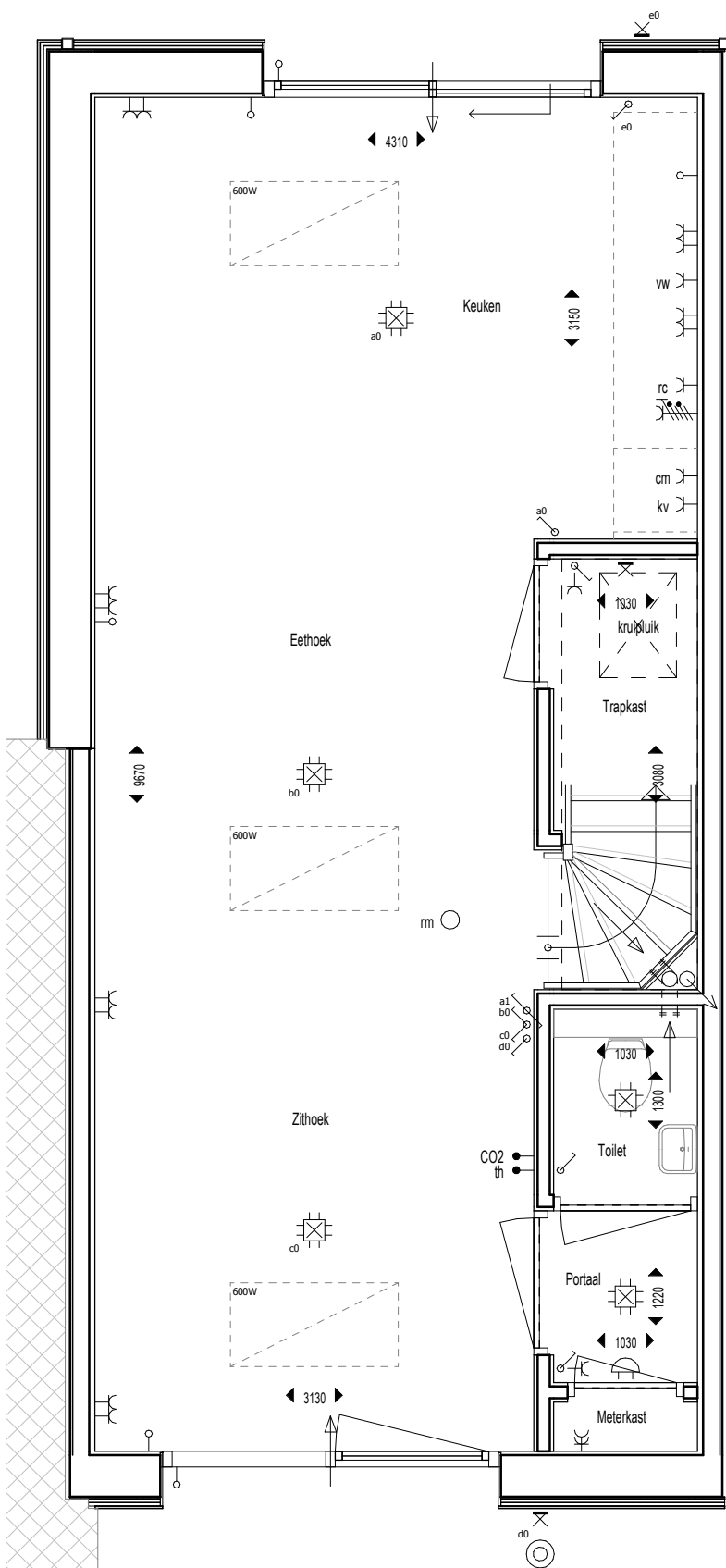
begane grond
