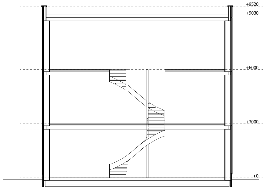
langsdoorsnede
