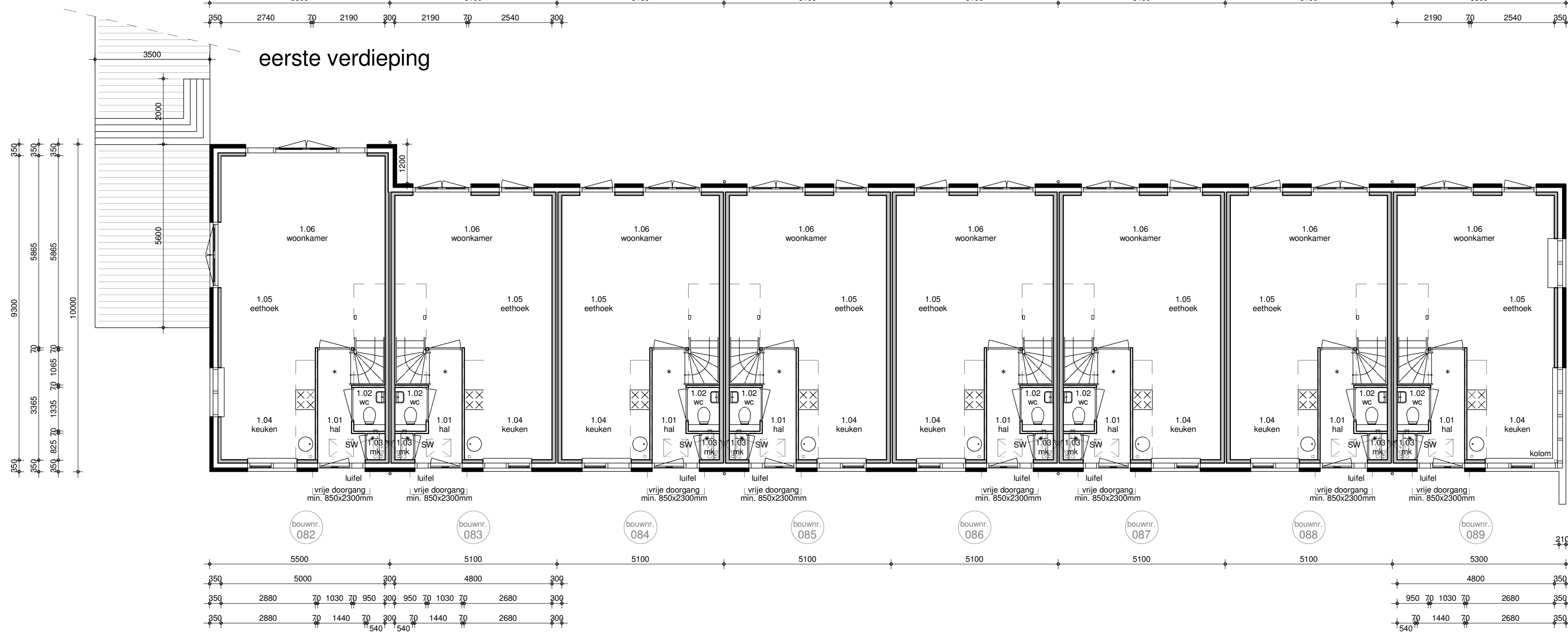
begane grond
