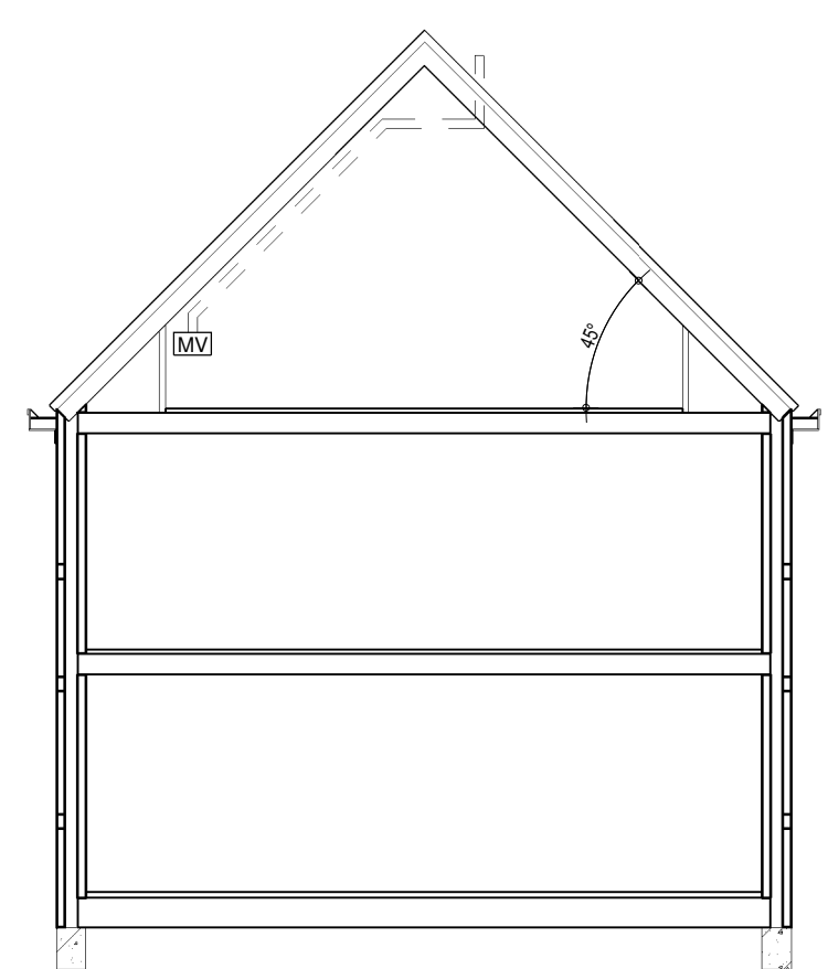
doorsnede
