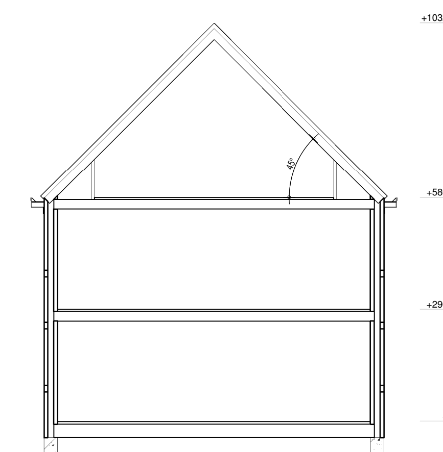
doorsnede
