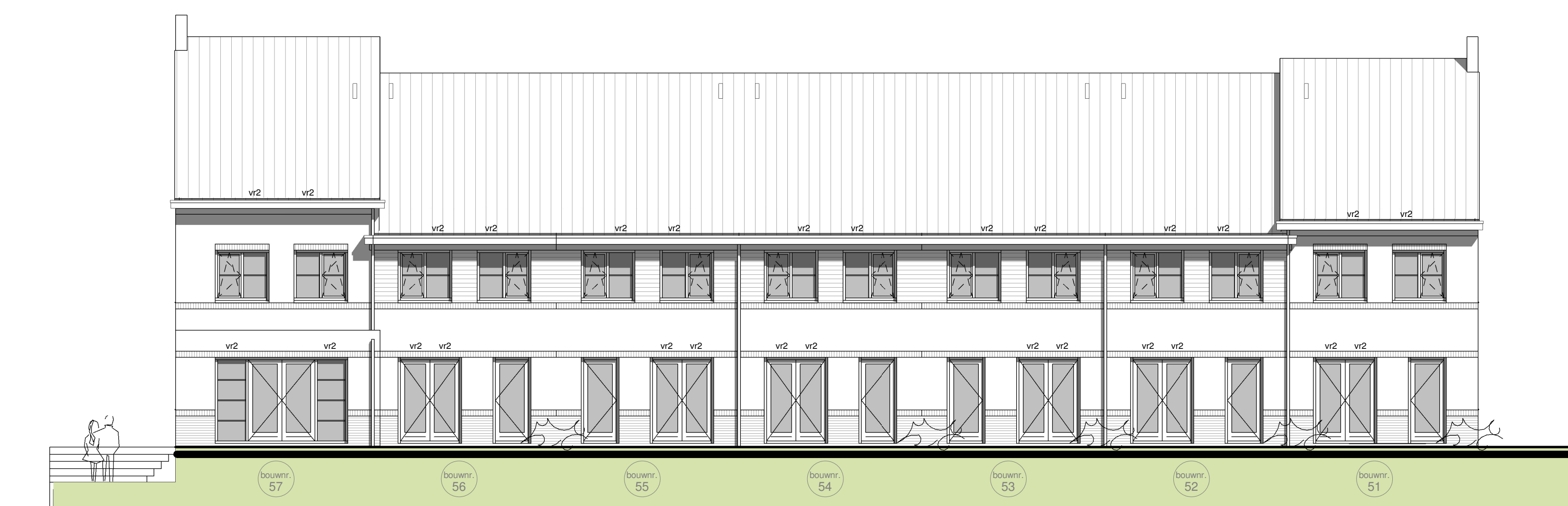
achtergevel
