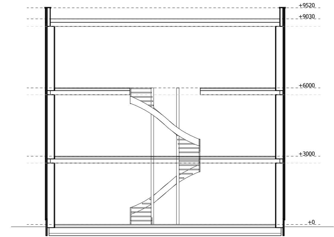
langsdoorsnede
