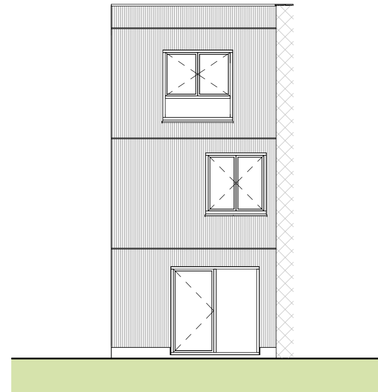
voorgevel
