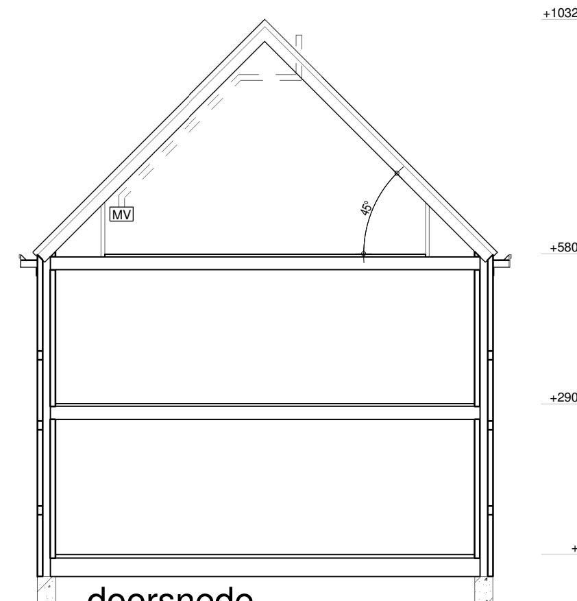
doorsnede
