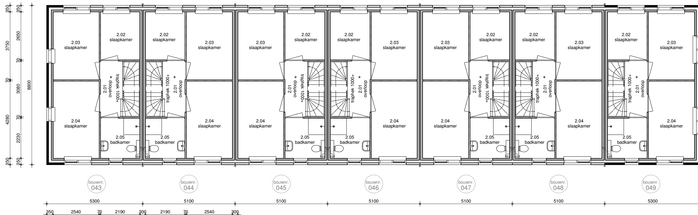
eerste verdieping
