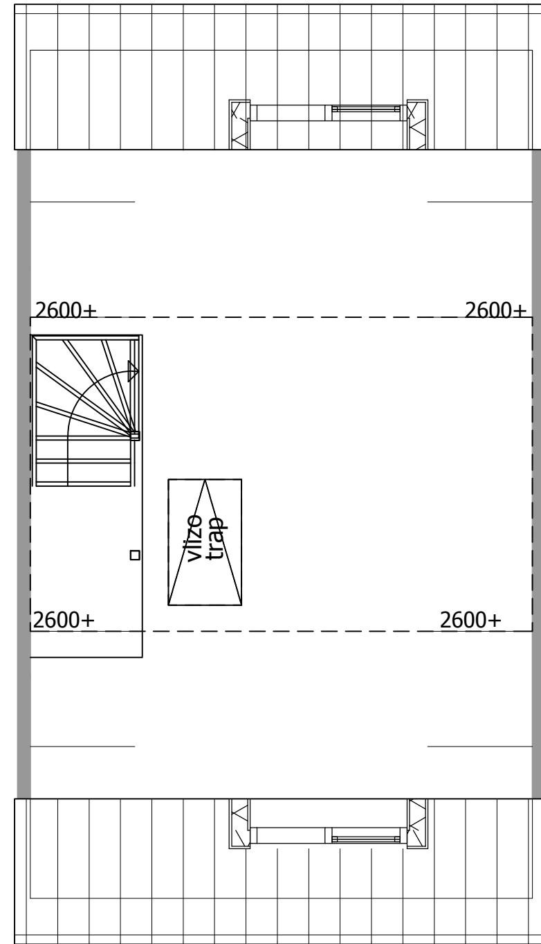
24.220 optie dakkapel
