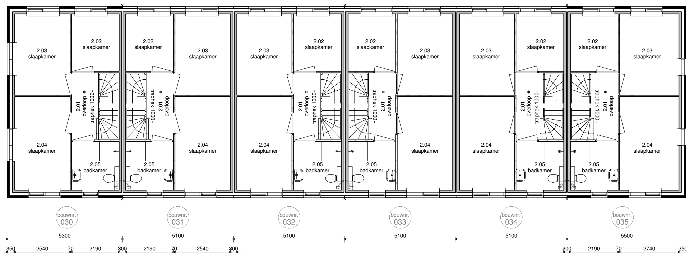
eerste verdieping
