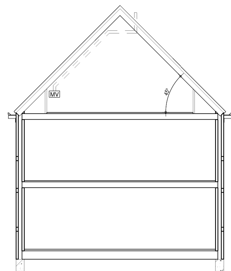
doorsnede
