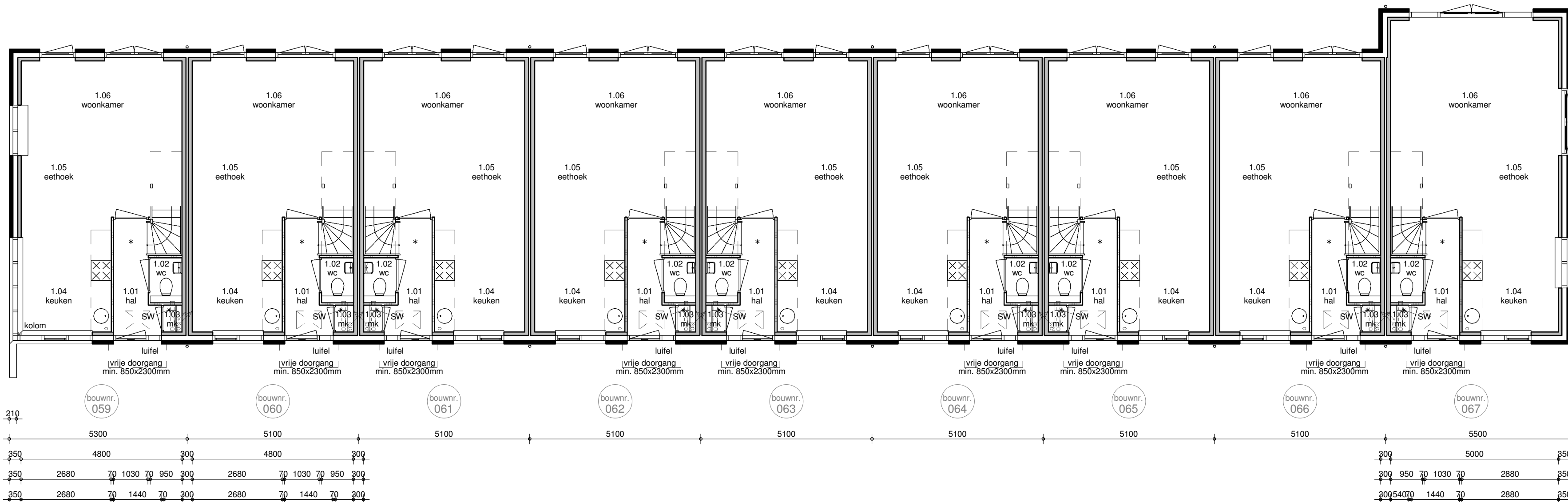
begane grond
