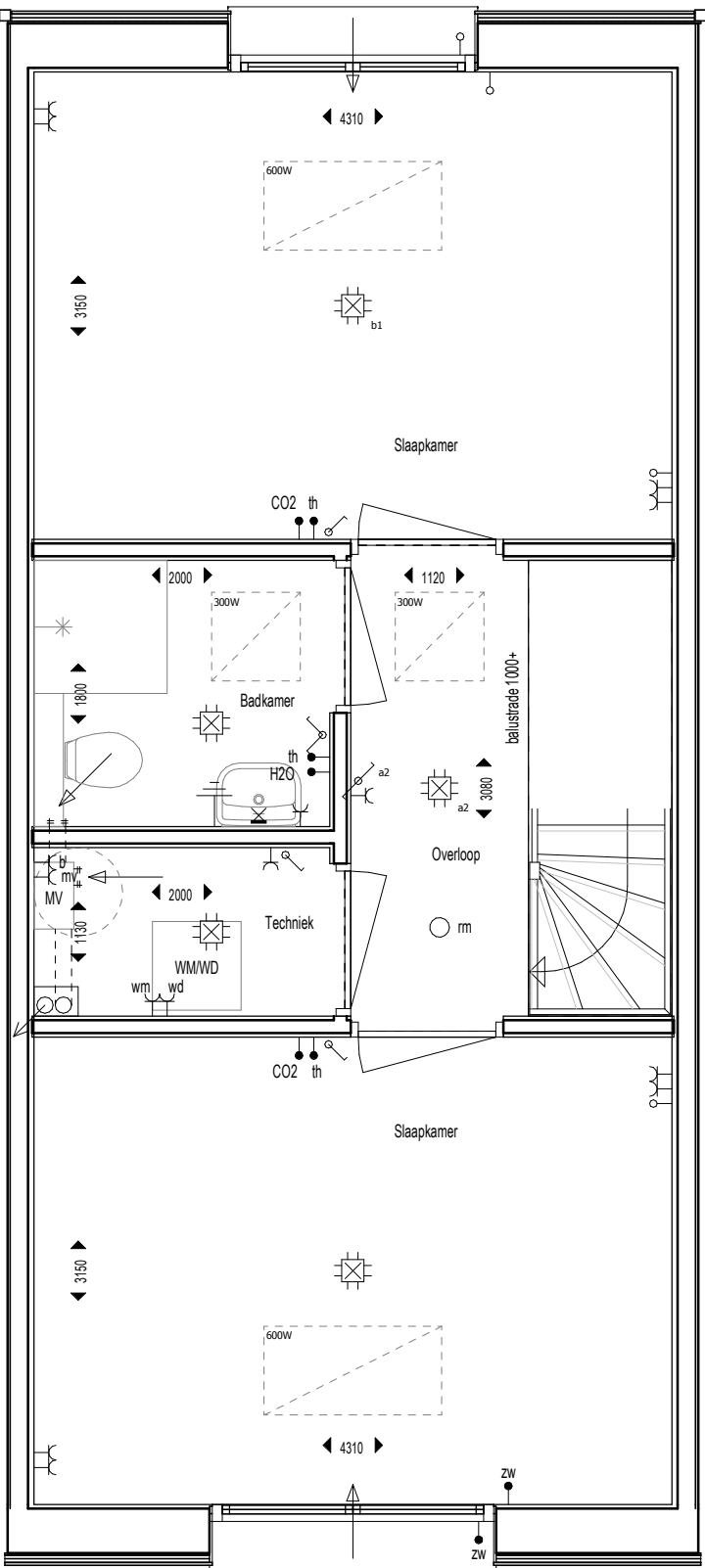
tweede verdieping
