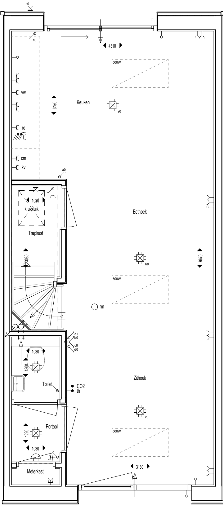
begane grond
