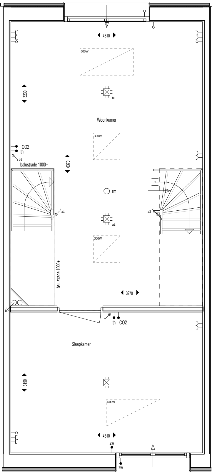
eerste verdieping
